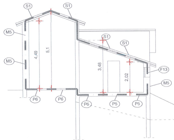
SEZIONE B-B FABBRICATO B
